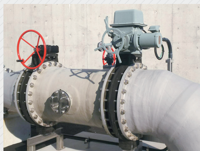
海水ライン(大口径バタフライ弁)
